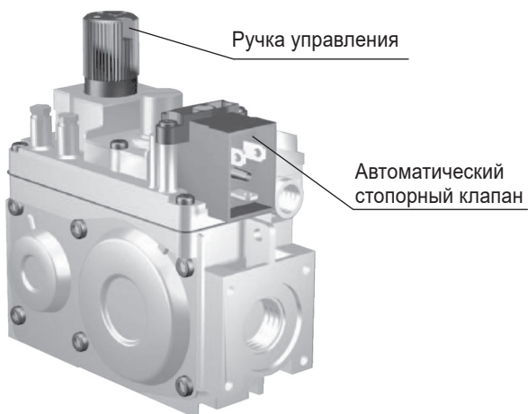
Рис. 5. Автоматика 820 нова
