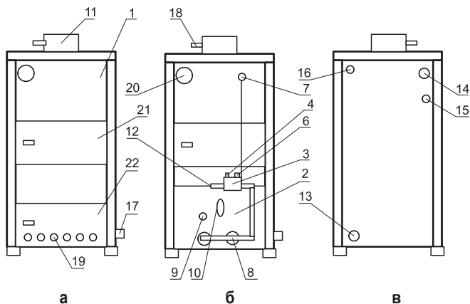
Рис. 1. Устройство котла
